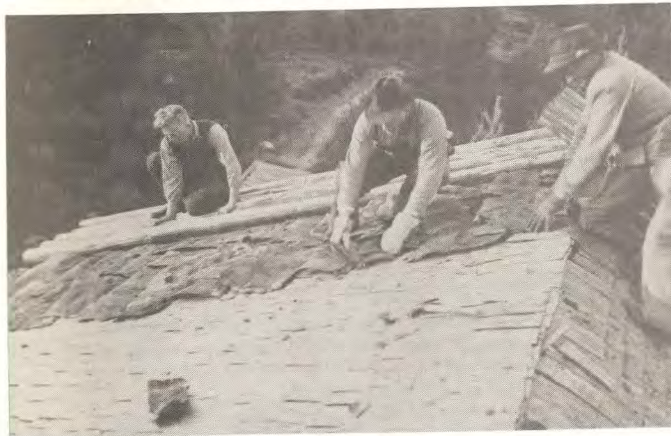
Figur 101. Näver- och vedtäckning på ett gammalt pärttak. Foto Norrbottens museum.
