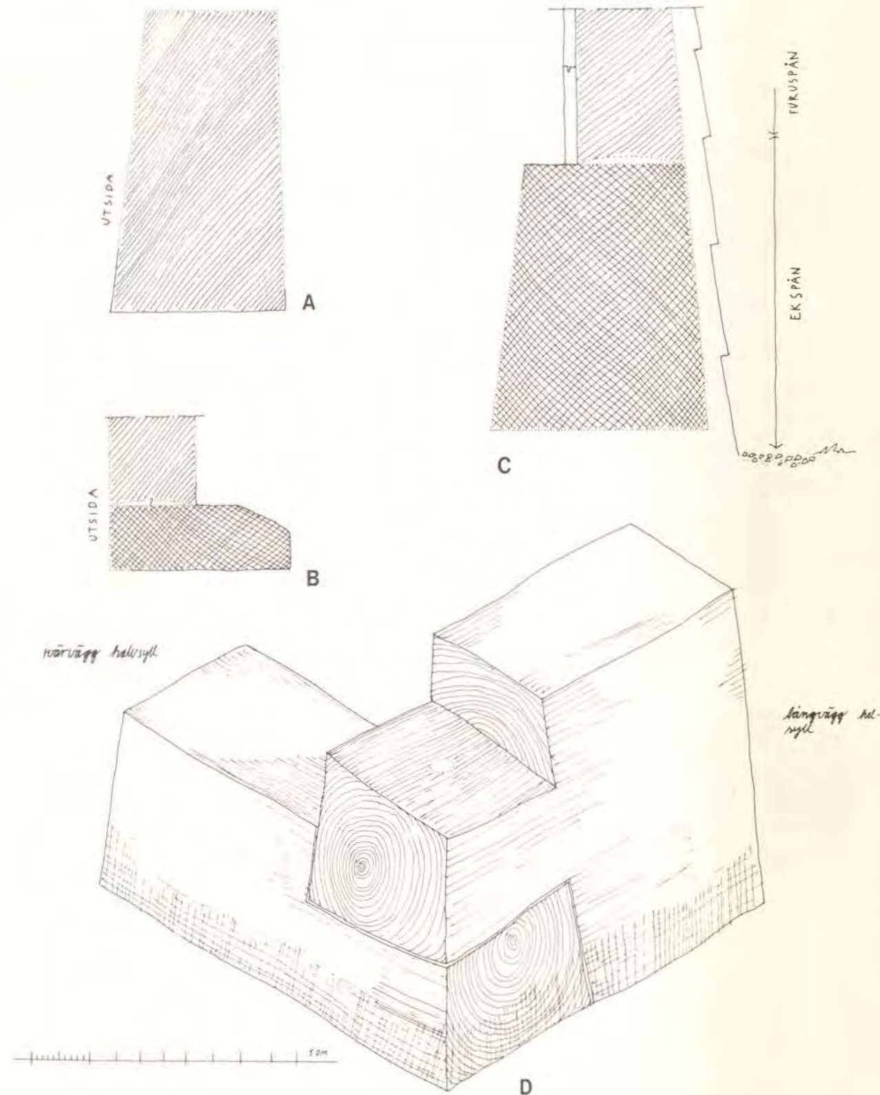
Figur 43. Syllar i timmerkyrkorna.
