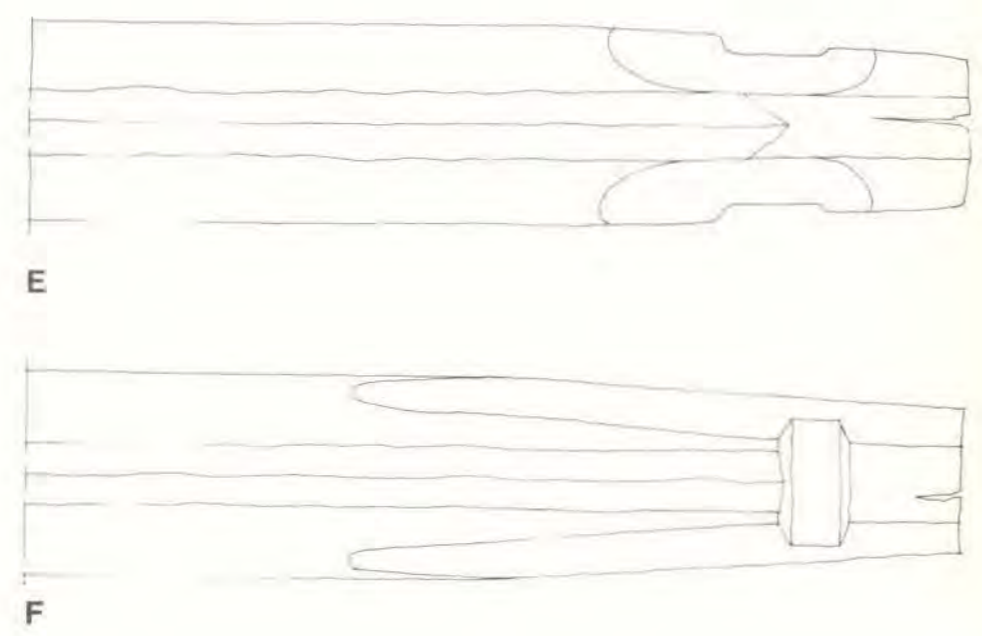
Figur 69. Drag. A. Dragets form i Dalarna. B. Dragets form i timmerkyrkorna. C. Principen för fogens tätning. D. Två timmervarv i dörrpartiet från Fåsås (1280-1290-tal), Zornmuseet, Mora. Uppmätning. E. Rännknutad stock där draget avslutas i knuten (sedd från undersidan). F. Stock med över- och underhugg (sedd från undersidan).
