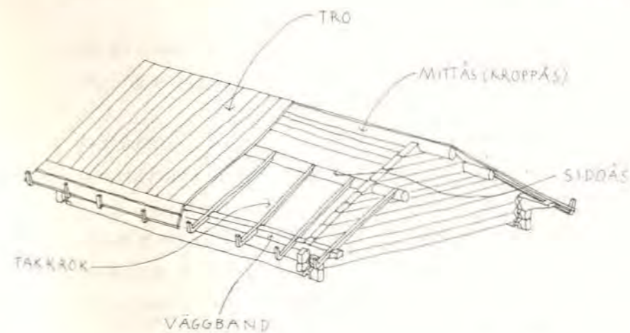
Figur 91. Åstak. Versal = principskiss. Gemen = verkningssätt. A. Mittås. B. Mittås och sidoåsar. C. Laggtak.
