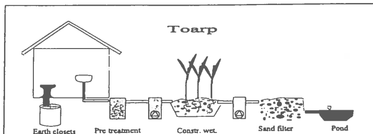
Figur 7. Ett avloppssystem för BDT-vatten. Exemplet är hämtat från Toarp (Kärman 1997).
