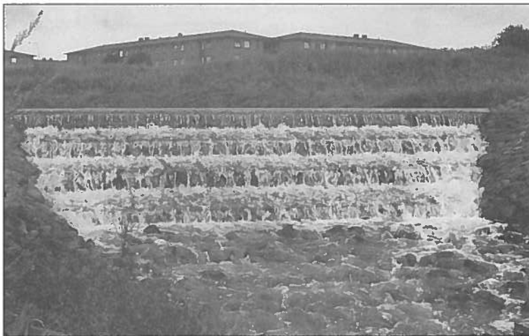
Figur 23. Överst ett trappstegsformat inlopp i form av ett vattenörag (Halmstad), och nederst ett trappstegsformat utlopp från en dagvattendamm (Mölndal). Foto: Jesper Persson.
