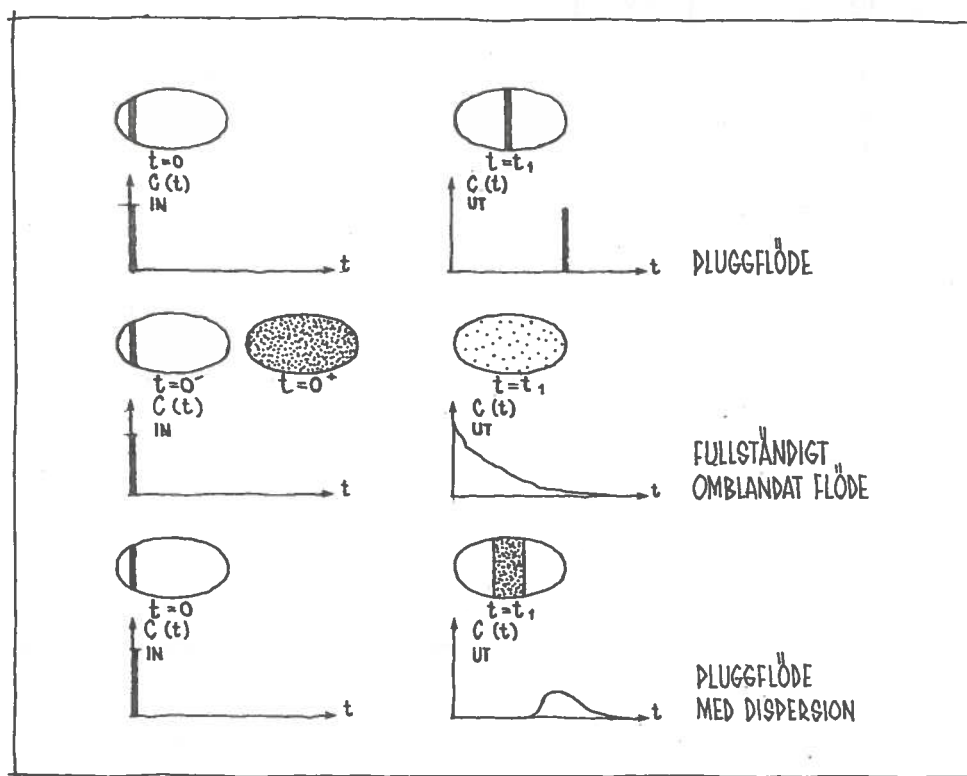
Figur 16. Exempel på pluggflöde, fullständigt omblandat flöde och pluggflöde med dispersion. Figurerna visar dels hur spårämnet sprider sig i planet och dels generella utseende på koncentrationsändringen i en punkt (vid utgående vattnet) med avseende på tiden, i de tre fallen.
