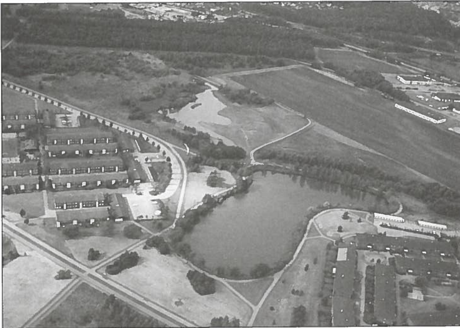
Figur 9. Vallås båda dammar som exempel på en djupare sedimentationsdamm (syns i förgrunden) som följs av en grundare vegetationsdamm. Sedimentationsdammen anlades under 1960-talet samtidigt som omgivande bebyggelse och syftade primärt till att utjämna dagvattenflödet. Vegetationsdammen tillkom 1992. Foto: Sven-Erik Jönsson.
