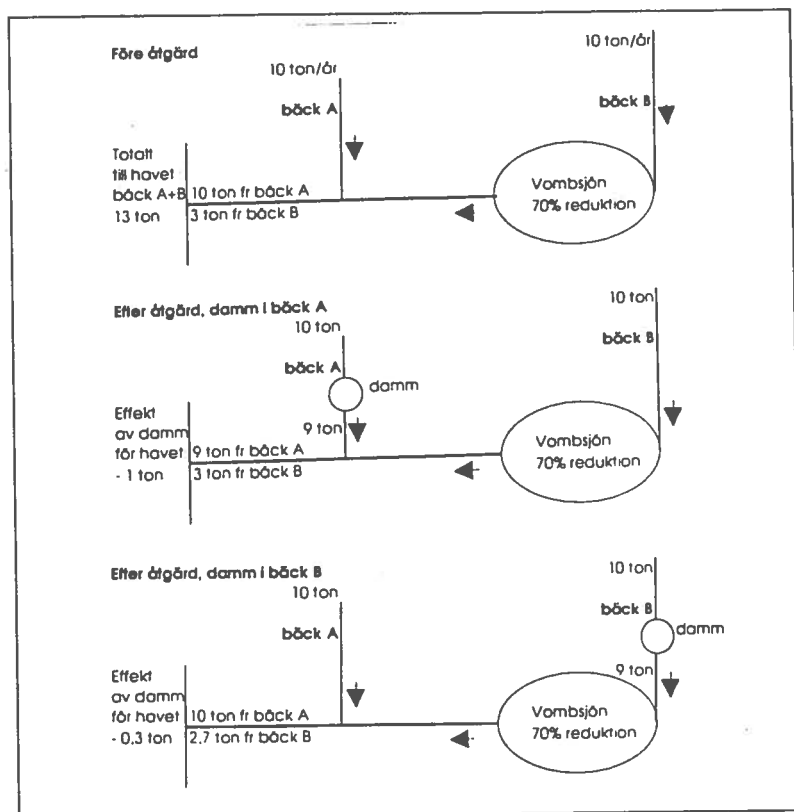
Figur 12. Ett exempel på effekten av en damm med avseende på dess placering i avrinningssystemet (Ekologgruppen 1993).
