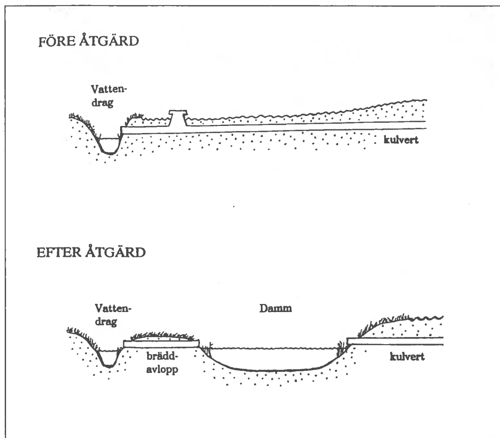
Figur 10. Kylvertdamm eller fångdamm i anslutning till utloppet från en kylvert (Ekologgruppen 1990).
