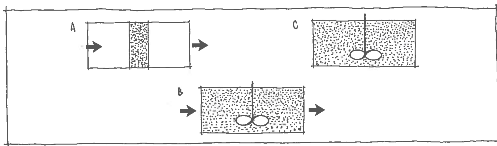
Figur 20. Tre ideala reaktionskärl, som visualiserar de två ideala flödestyperna pluggflöde och fullständigt omblandat flöde. a) Pluggflödeskärl med pluggflöde, b) fullständigt omblandat kärl med fullständigt omblandat flöde och c) slutet reaktionskärl utan in- och utflöde.
