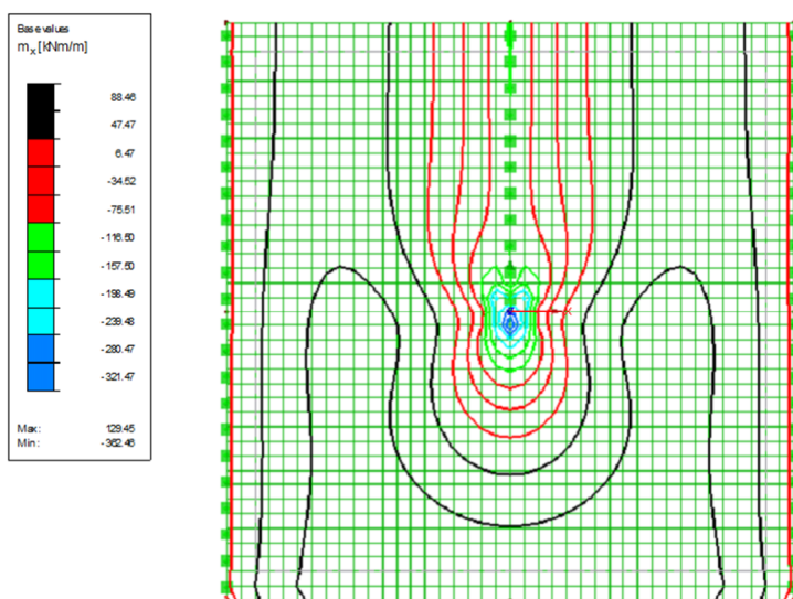
Figur 3.3.1.3 Böjmoment m_x , mindlinelement 0,5 \times 0,5 m.
