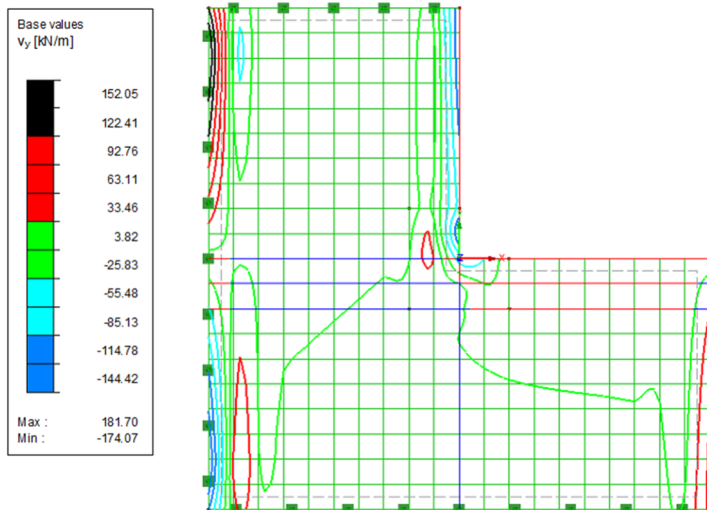
Figur 4.7.7 Tvärkraftsplan v_y . Fri kant ovanför hörn bär uppåt i figuren (negativ). Den högra fria kanten bär nedåt i figuren (positiv).
