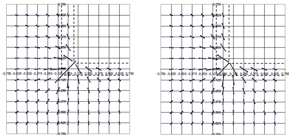
Figur 4.6.2.2a och b Huvudvärkrafter kring det inre hörnet, till vänster fast inspänt upplag och till höger elastiskt inspänt upplag, samma skala.
