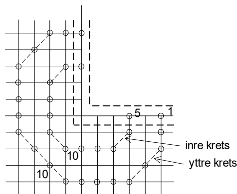
Figur 4.6.2.3 Redovisningspunkter för huvudvärkraft runt inre hörn, rutnät 0,125 m.
