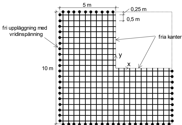
Figur C.3.1 Balkrostmodell.
