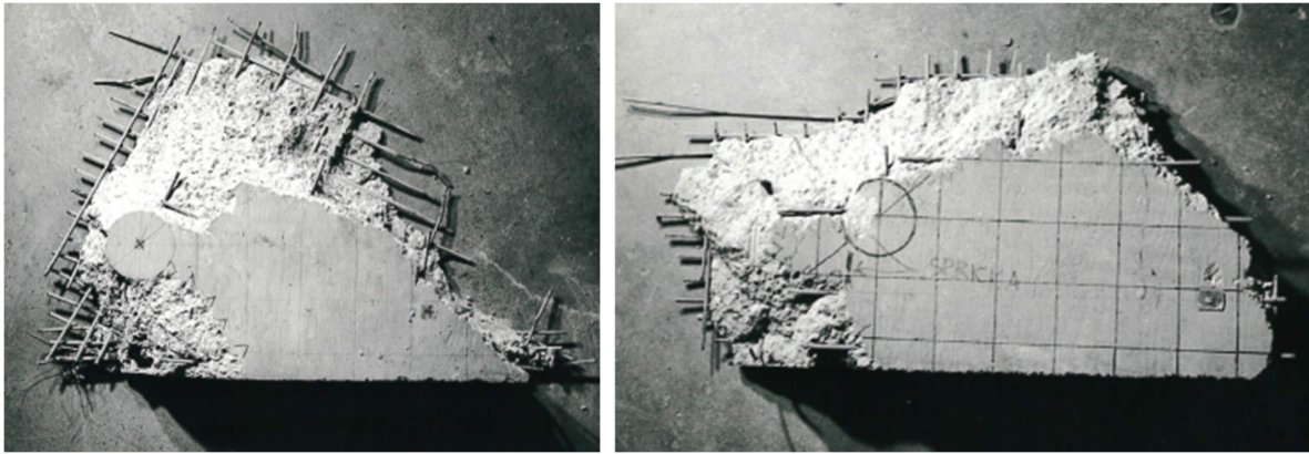
Figur 4.3.2.6a och b Urtagna "stanskoner" ur 50^\circ snedvinkliga tvåspansn plattor; i resp bild är trubbigt hörn till vänster och spetsigt till höger; centrisk stödreaktion; Hallbjörn (1968).
