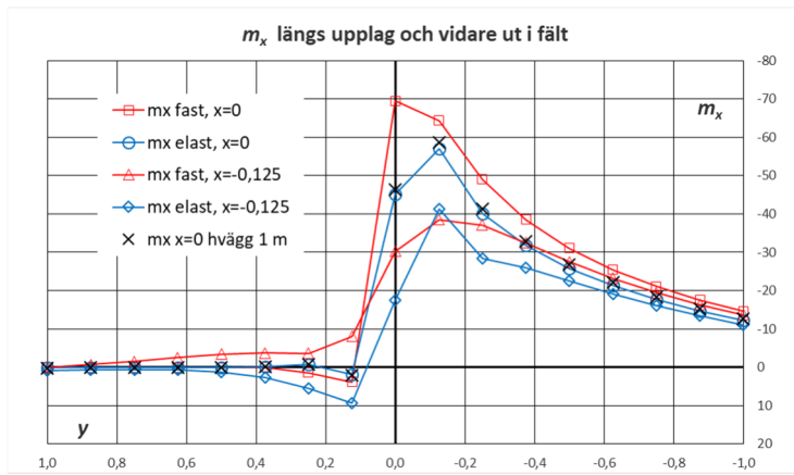
Figur 3.5.2.1 Jämförelse av m_x längs upplag (vänstra delen) och vidare ut i fält, x = 0 , samt längs näraliggande snitt x = -0,125 . Elastiska resp fasta linjeupplag.
