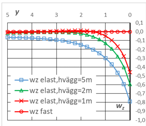
Figur 4.4.4.5 Nedböjning (mm) längs upplag vid vägghöjd 5,0, 2,0 och 1,0 m. Figur 4.4.4.6 Upplagsreaktion (kN/m) längs upplag vid vägghöjd 5,0, 2,0 och 1,0 m.
