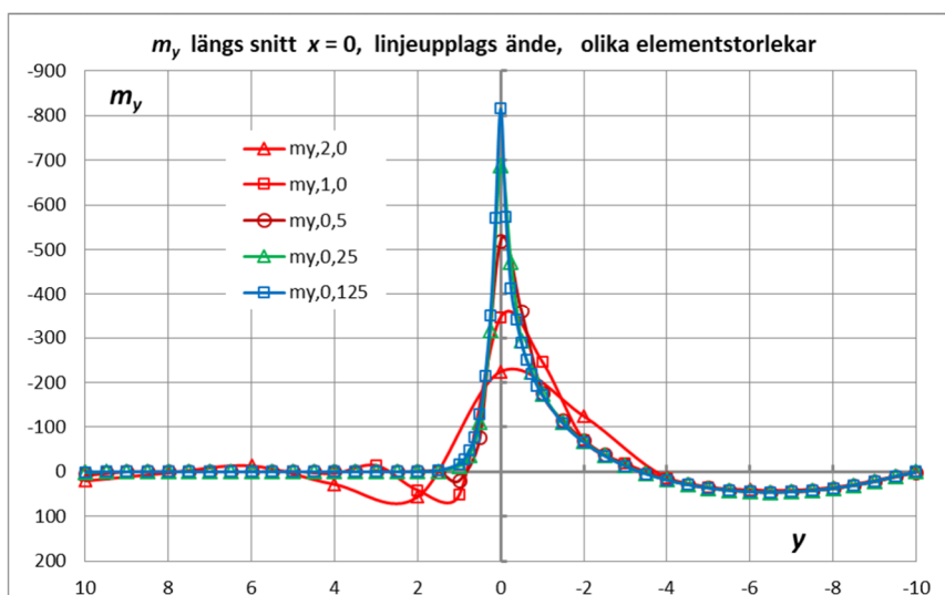
Figur 3.3.1.6 m_y längs snitt x = 0 .
