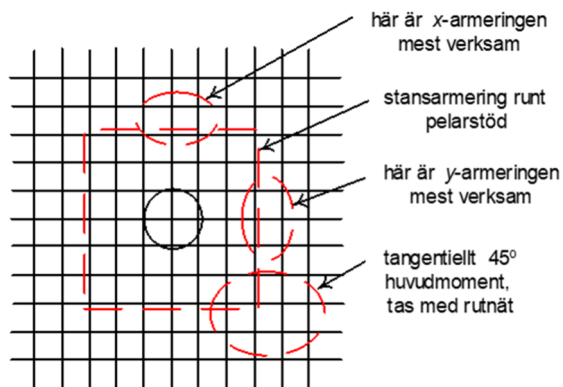
Figur A.1.1 Pelarstöd.
