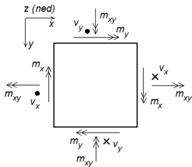
Figur 2.1.4 Positiva storheter. Figur 2.1.5 Sam- och motverkan vid fria kanter.
