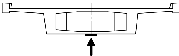
Figur 4.8.2 Sektion.
