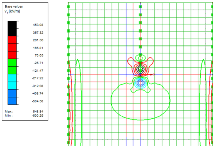
Figur 4.4.1.5 Tvärkraftsplan v_y , bärning i riktning nedåt i figuren räknas som positiv, mindlinelement 1,0 x 1,0 m.
