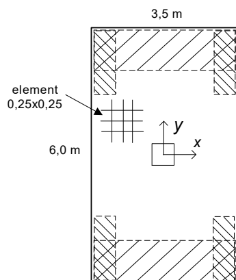
Figur 4.8.6 Beräkningsmodell, plan.
