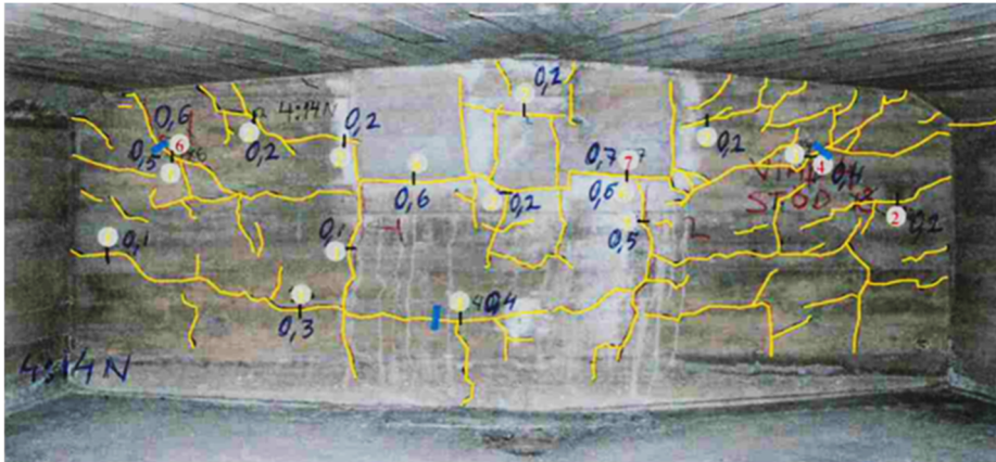
Figur 4.8.5d Sprickbild tvärbalk 4.14 norra.
