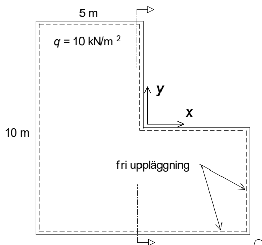
Figur 4.5.1.1 Studerad platta.
