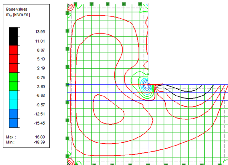
Figur 4.7.3 Momentplan m_x , mindlinelement 0,5 \times 0,5 \text{ m} . Obs negativa moment vid inre hörn.
