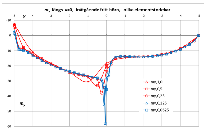
Figur 3.4.5 m_y längs snitt x = 0 .
