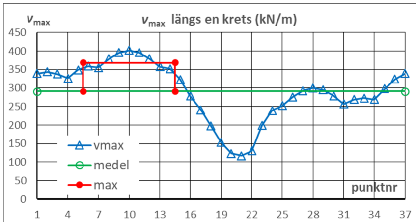
Figur A.4.1 Bestämning av tilläggfaktör vid stansningsberäkning.
