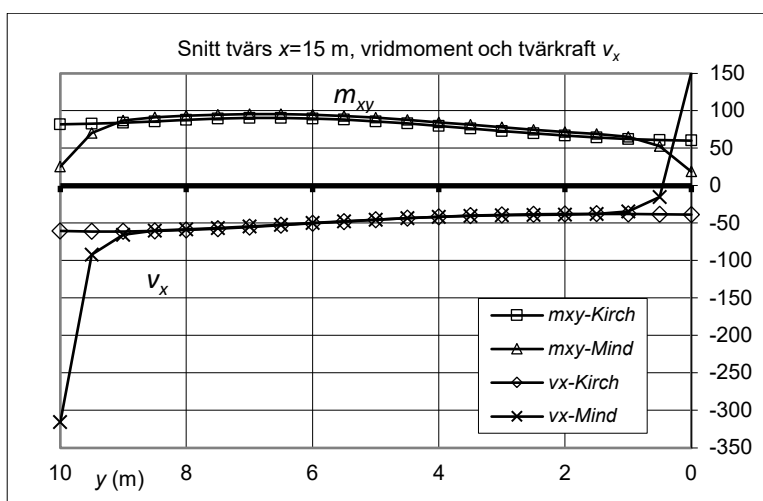
Figur 2.4.4 Jämförelse av vridmoment och tvärkraft v_x i snitt x=15 m med kirchoff- resp mindlinelement.
