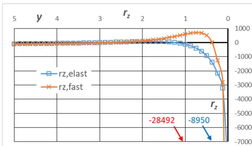
Figur 4.4.4.1 Upplagsreaktion längs stödlinjen, element 0,125 m.
