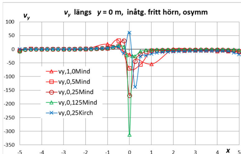
Figur 4.7.9 Tvärkraft v_y (kN/m) längs y = 0 m (x-axeln). De lokala variationerna vid sidan om hörnet avtar vid finare elementindelning.
