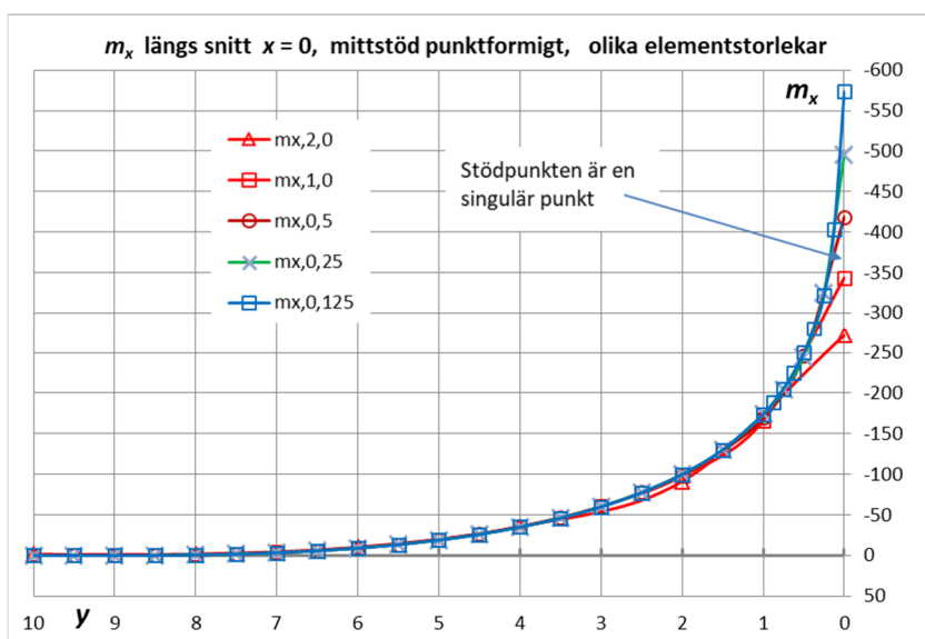
Figur 3.2.1.4 m_x vid punktupplag (tangentiellt moment), toppmomentet ökar utan begränsning vid allt finare elementindelning.
