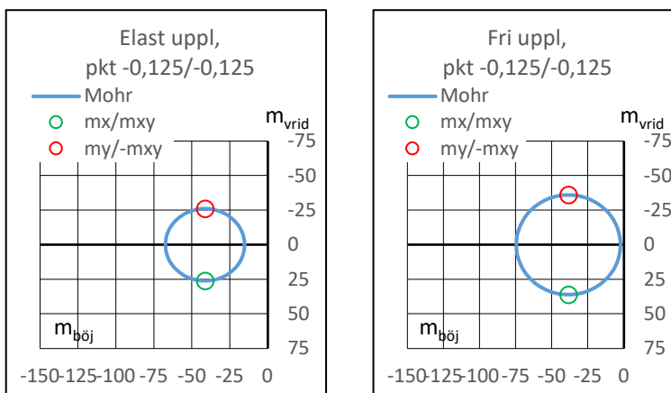
Figur 3.5.2.5 Momenttillstånd visat med Mohrs cirkel.
