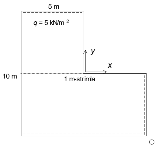
Figur 3.4.6 1 m-strimla.
