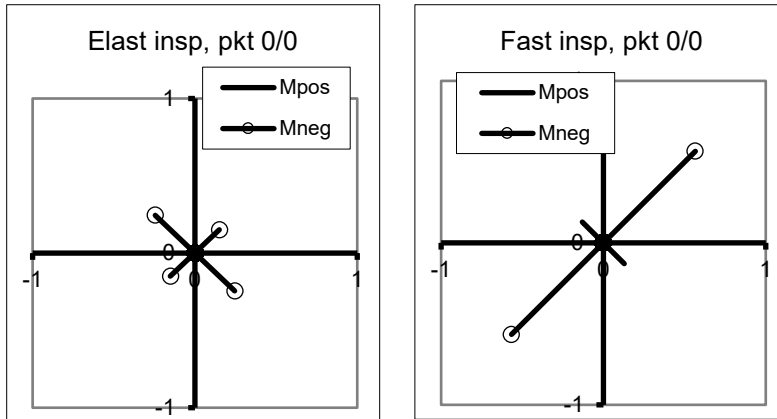
Figur 3.6.2.2 Huvudmoment i inre hörn, samma skala, element 0,125 (x-axel åt höger).
