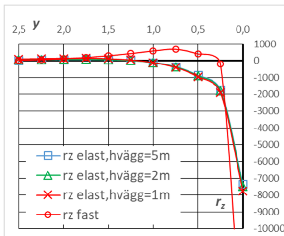
Figur 4.4.4.5 Nedböjning (mm) längs upplag vid vägghöjd 5,0, 2,0 och 1,0 m. Figur 4.4.4.6 Upplagsreaktion (kN/m) längs upplag vid vägghöjd 5,0, 2,0 och 1,0 m.
