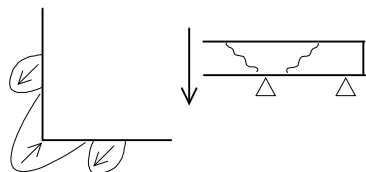
Figur 4.5.1.5 Tendens till skjvsprickor nära hörn.
