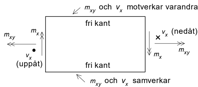
Figur 2.1.4 Positiva storheter. Figur 2.1.5 Sam- och motverkan vid fria kanter.
