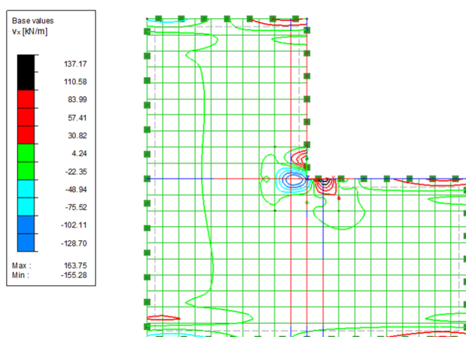
Figur 4.5.1.4 Tvärkraftsplan v_x , bäring i riktning mot vänstra upplaget räknas som positiv, mindlinelement 0,5 x 0,5 m.
