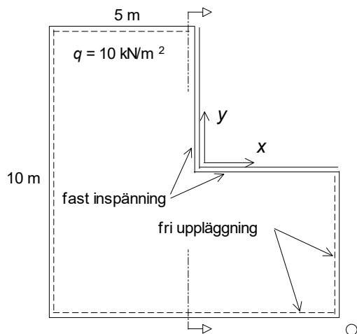
Figur 3.6.1.1 Studerad platta.
