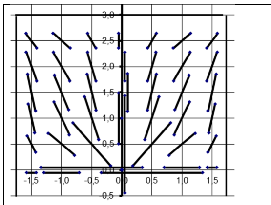
Figur 4.8.9 Huvudtvärkrafter i halva plattan, gles redovisning.
