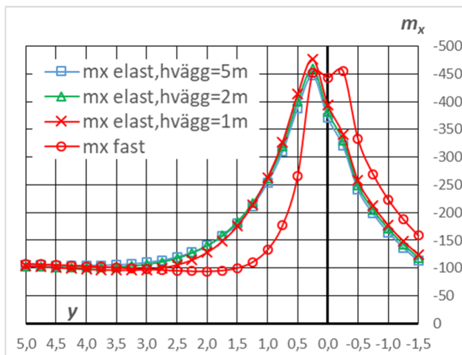
Figur 4.4.4.7 Bøjmoment m_x (kNm/m) i plattan längs upplagslinjen och ut i fält.
