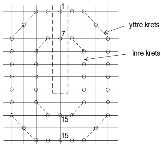
Figur 4.4.4.3 Redovisningspunkter för huvudvärkraft runt stödände, element 0,125 m.
