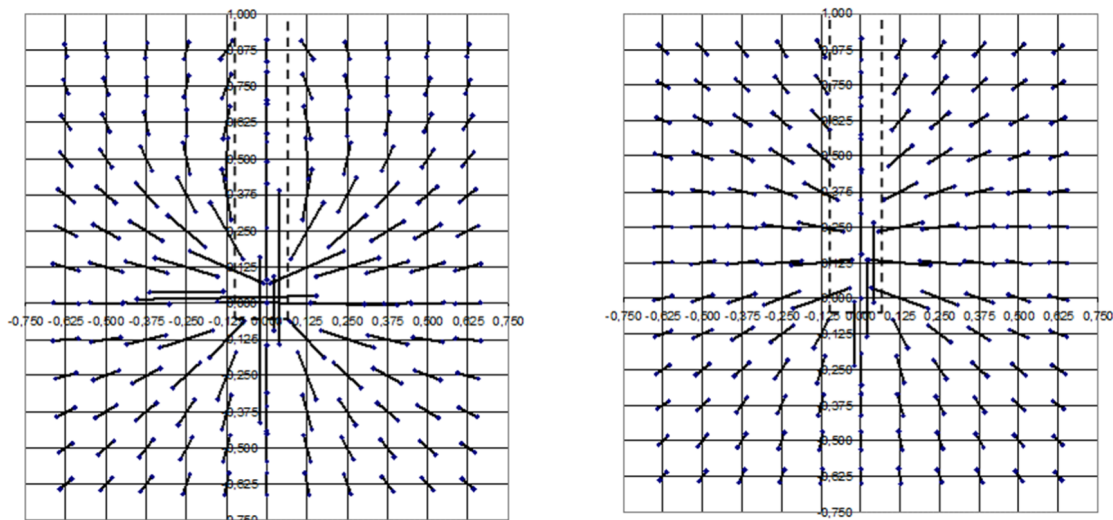
Figur 4.4.4.2a och b Huvudvärkrafter kring stödslutet, till vänster fast upplag och till höger elastiskt upplag, samma skala, element 0,125 m. Några tvärkraft-symboler är sidoförskjutna för tydlighets skull.
