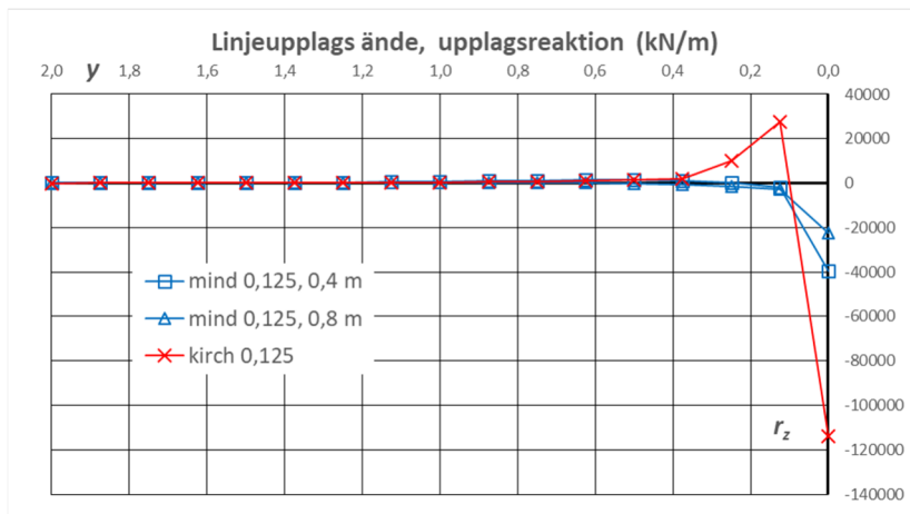
Figur 4.4.3.1 Upplagsreaktion längs del av linjeupplag, med mindlin- och kirchoffelement.
