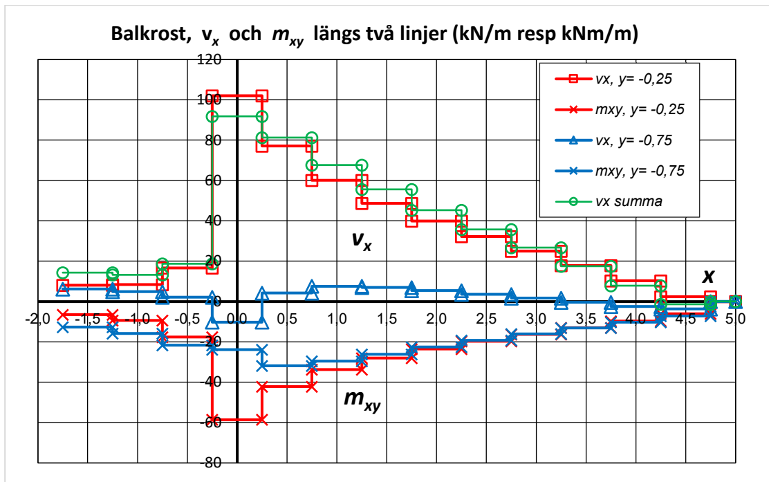
Figur C.6.2 Balkrost, tvärkraft och vridmoment i x -balkar ( kN/m resp kNm/m ), positiva värden uppåt.
