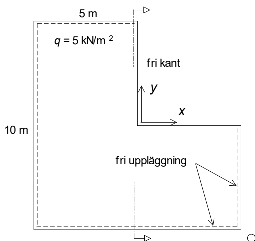
Figur 3.4.1 Studerad platta.
