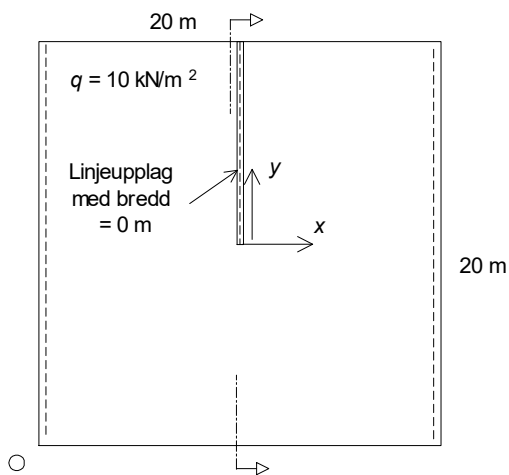
Figur 3.3.1.1 Studerad platta.
