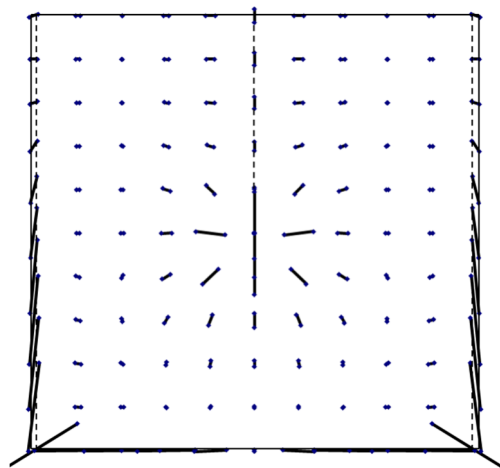
Figur 4.4.1.2 Huvudtvärkrafter, mindlinelement 0,5 \times 0,5 m, gles redovisning.
