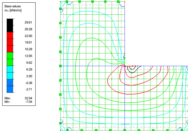
Figur 3.4.3 Böjmoment m_x , mindlinelement 0,5x0,5 m.
