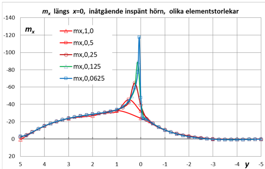
Figur 3.6.1.5 m_x längs snitt x = 0 .
