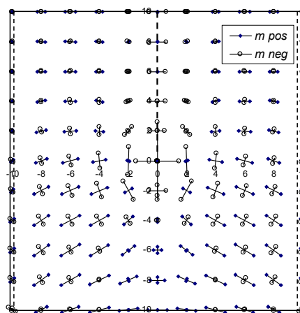
Figur 3.3.1.2 Huvudmoment, mindlinelement 0,5 \times 0,5 m, gles redovisning.
