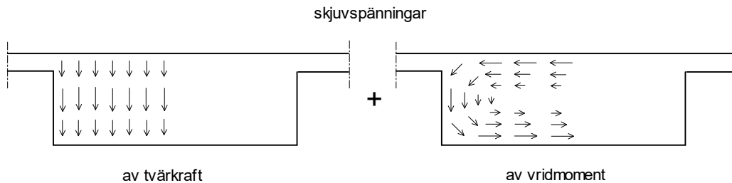
Figur 2.1.1 Skjuvspänningar vid plattkant vilka ger tvärkraftens "basvärde" (kN/m, vänstra delfiguren) resp "kantillskott" (kN, högra delfiguren).
