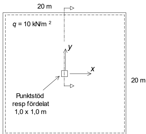
Figur 3.2.1.1 Studerad platta.
