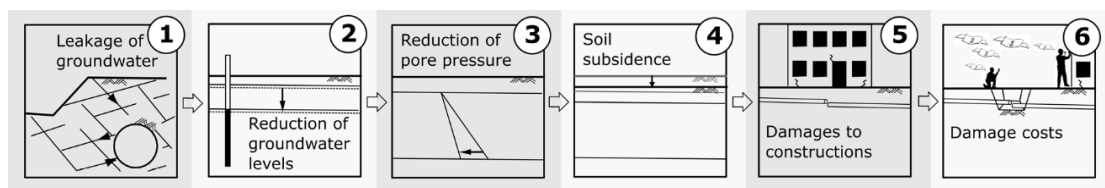
Figur 2. Händelsekedjan för skador på anläggningar till följd av bortledning av inläckande grundvatten till en undermarksanläggning (från Sundell (2018)).
