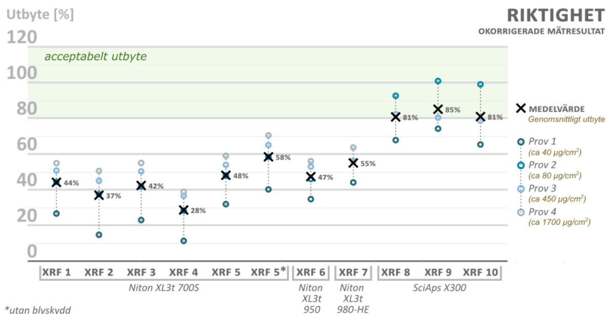
Figur 12. Beräknade utbyten för fyra olika färgprov (prov 1–4, Undersökning 2) för de utvärderade XRF-instrumenten kalibrerade i \mu\text{g}/\text{cm}^2 . Notera att inga resultat kunde redovisas för prov 4 för instrumenten av modell SciAps X300 då dessa instrument ej anger halter som överskrider ca 600 \mu\text{g}/\text{cm}^2 . De redovisade medelvärdena (x) är således beräknade utifrån fyra prov för XRF 1–7 och från tre prov för XRF 8–10. Den gröna rutan visar kriteriet för acceptabelt utbyte (80–120%).
