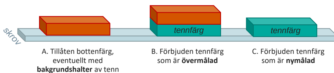
Figur 4. Illustration av de tre huvudsakliga scenarios som kan förekomma på en båt med tennorganisk färg på ett skrov.
