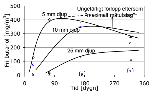
Figur 20 Koncentration i betongen.
