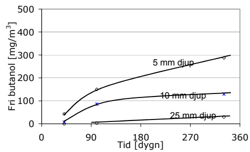
Figur 24 Koncentration i betongen.
