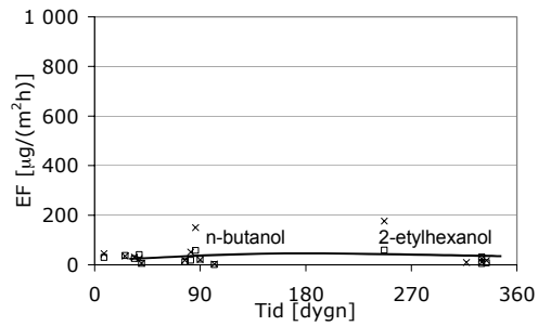
Figur 37 Emission från ytan.
