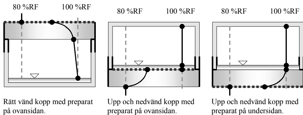
Figur 8 Fuktfordelningen vid de tre olika positioner av betongpuck och spärnskikt som användes hos kopporna i studien. Ytövergångsmotstånd har försumrats.
