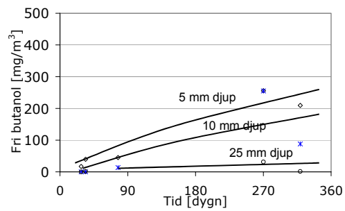
Figur 32 Koncentration i betongen.
