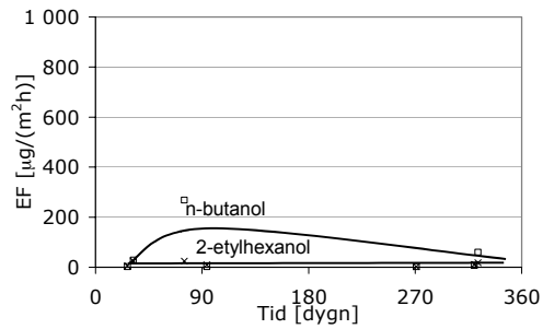
Figur 29 Emission från ytan.
