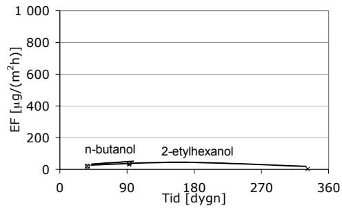
Figur 25 Emission från ytan.
