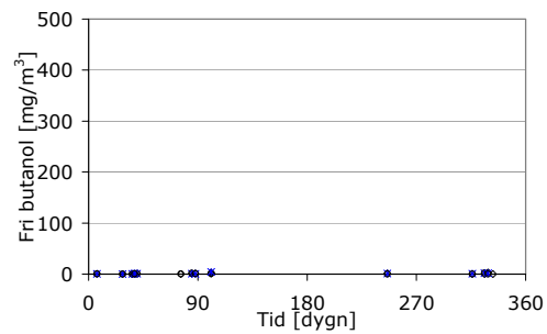
Figur 40 Koncentration i betongen.
