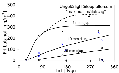
Figur 19 Koncentration i betongen.
