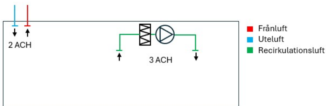
Figur 9. Principskiss för lokal recirkulationsluft i rum. Angivna luftväxlingar är endast exempel.
